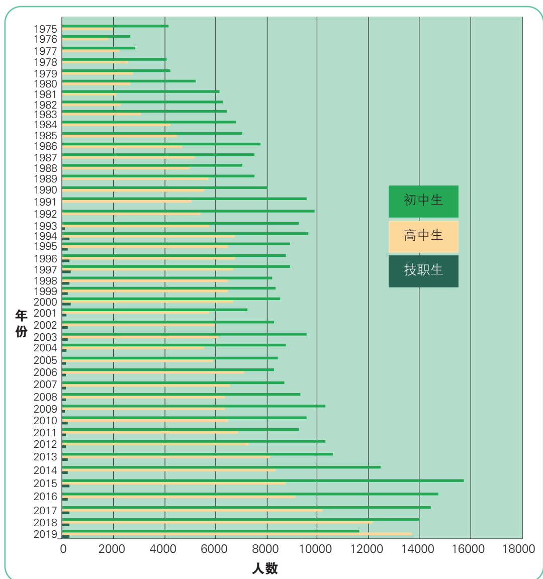
图表2：1975年至2019年历届统考考生人数统计图
